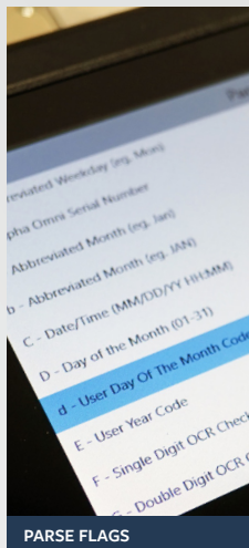
PARSE FLAGS
